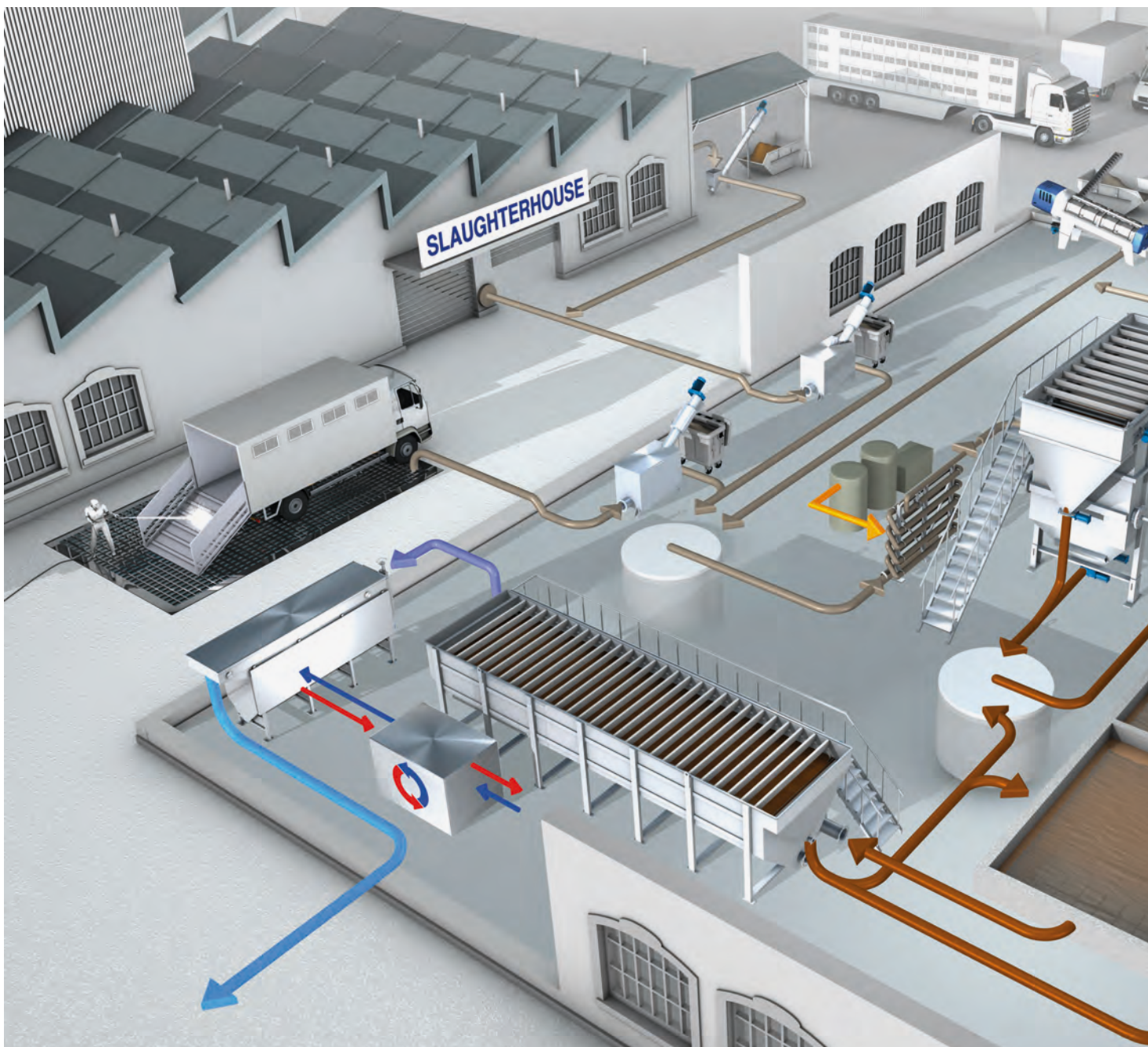
Maschinen und Einsatzgebiete der HUBER-Maschinenteknik im Abwasserprozess der Fleischindustrie.
